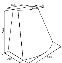
Jøtul I 400 narrow canopy
