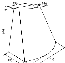
Jøtul I 400 wide canopy
